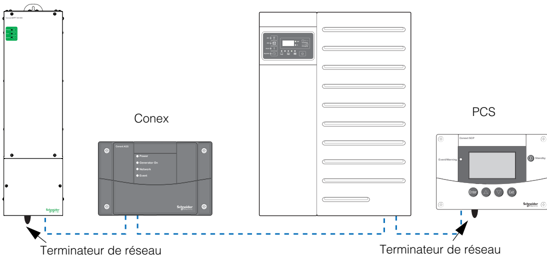
Figure 2-25 Exemple de réseau Xanbus
