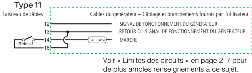
Figure 2-19 Type 11, Schéma de connexions
