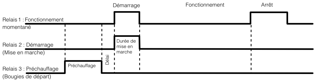
Figure C-8 Schéma de temporisation du mode MomentaryRun
