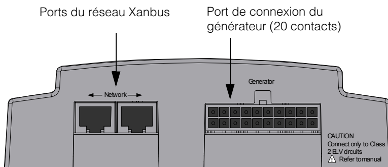
Figure 1-3 Conext AGS Partie inférieure
