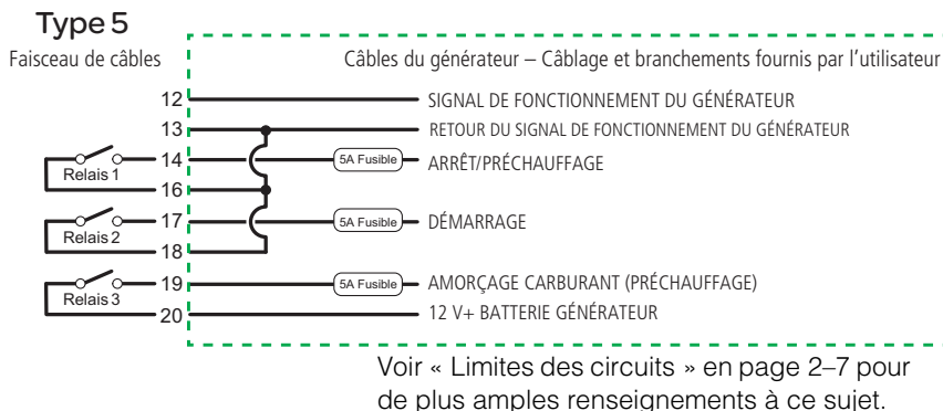
Figure 2-11 Type 5, Schéma de connexions
