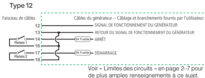
Figure 2-20 Type 12, Schéma de connexions
