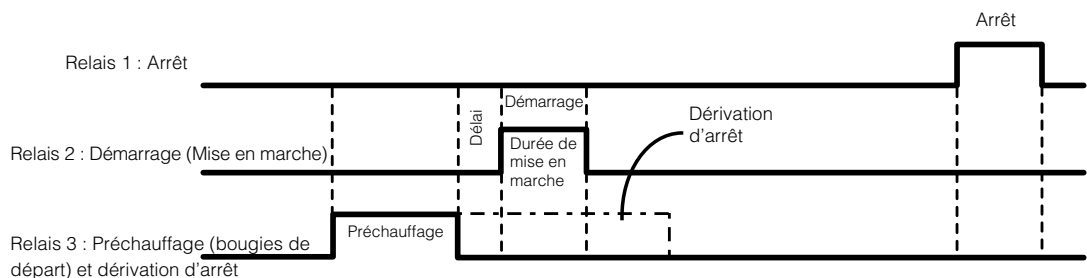
Figure C-10 Schéma de temporisation du mode StartStop
