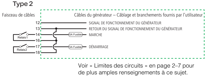
Figure 2-8 Type 2, Schéma de connexions
