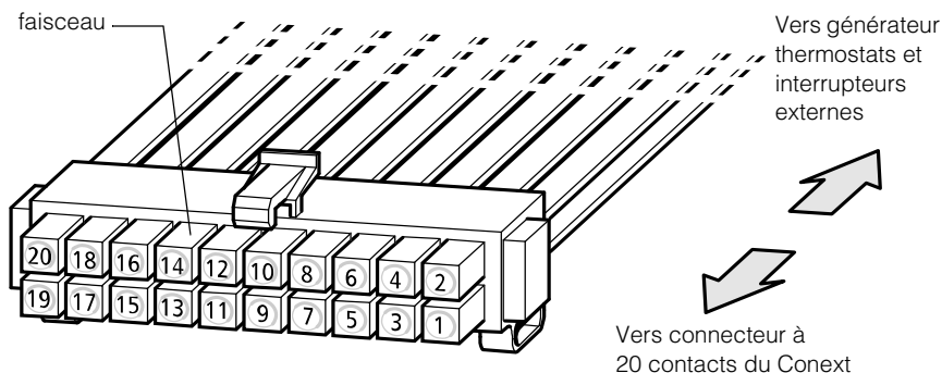
Figure 2-6 Conext AGS Faisceau de câbles
