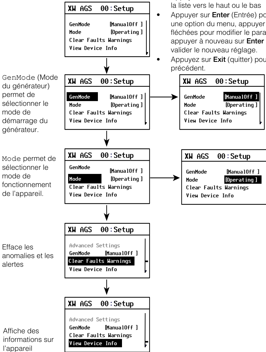
Figure 3-31 Arbrescence des menus des paramètres de base de l'Conext AGS
