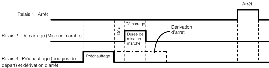
Figure C-11 Schéma de temporisation du mode PulseStop
