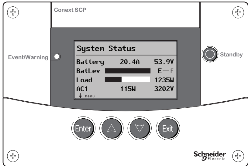
Figure 3-28 Écran d'état du système du PCS et touches de navigation
