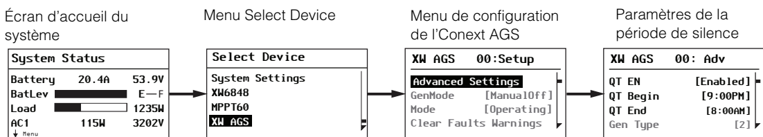
Figure 4-3 Utilisation de la fonction Quiet Time (période en repos)
