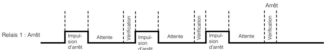
Figure C-12 Comportement du relais 1 en mode PulseStop
