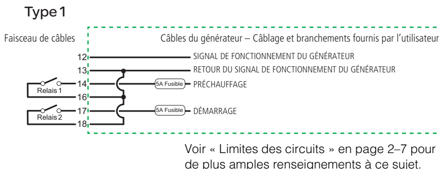
Figure 2-7 Type 1, Schéma de connexions
