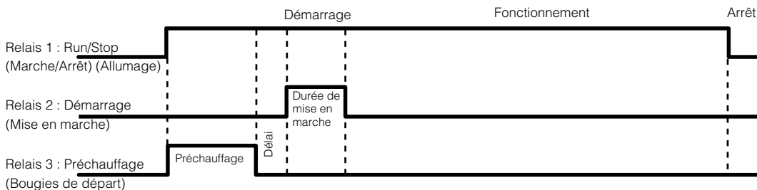
Figure C-7 Schéma de temporisation RunMode
