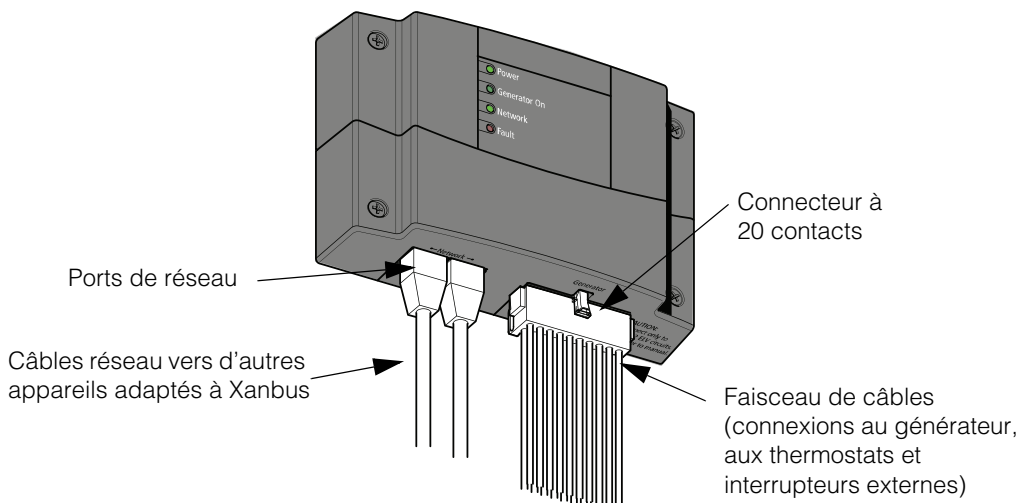
Figure 2-5 Connexions externes de l'Conext AGS
