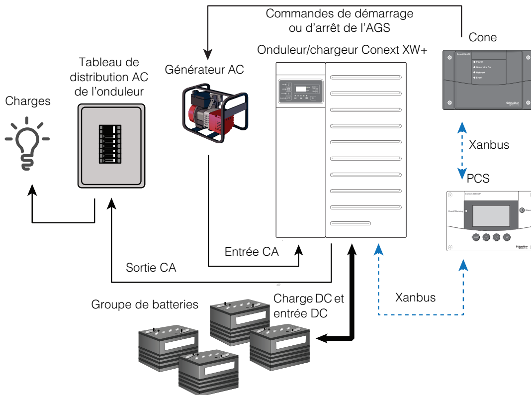
Figure 1-1 Fonctions de base de l'AGS Conext
