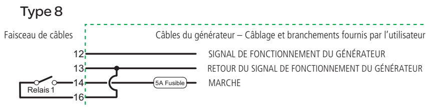
Figure 2-15 Type 8, Schéma de connexions (deux fils)
