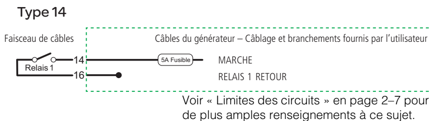
Figure 2-22 Type 14, Schéma de connexions (deux fils)
