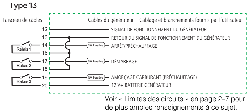
Figure 2-21 Type 13, Schéma de connexions
