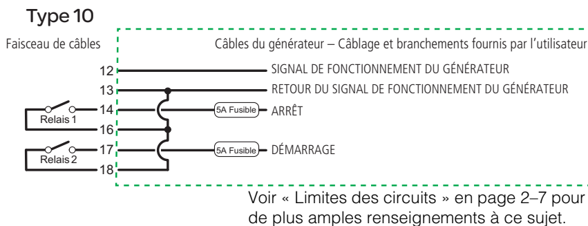
Figure 2-18 Type 10, Schéma de connexions
