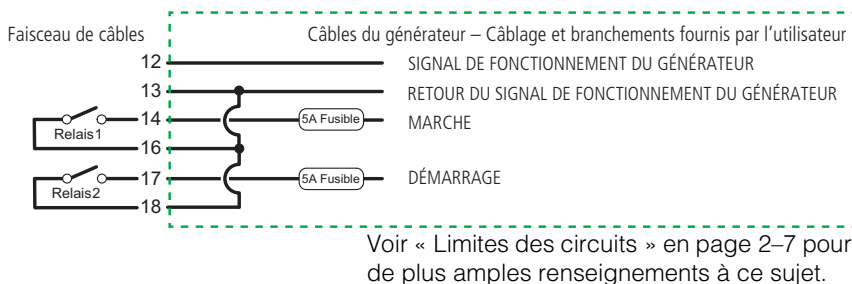
Figure 2-14 Type 7, Schéma de connexions (trois fils)
