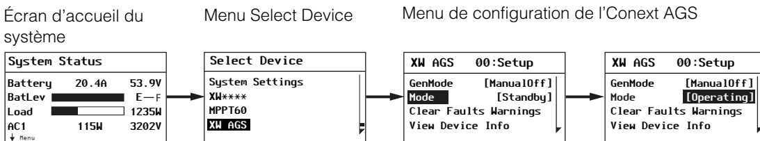
Figure 4-5 Rétablissement du fonctionnement de l'AGS
