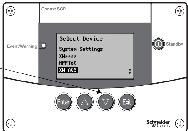
Figure 3-29 Affichage du menu Setup (Configuration) de l'AGS
