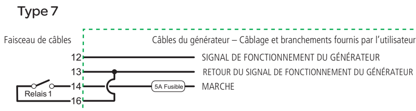
Figure 2-13 Type 7, Schéma de connexions (deux fils)
