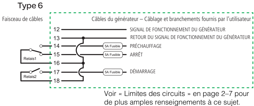
Figure 2-12 Type 6, Schéma de connexions
