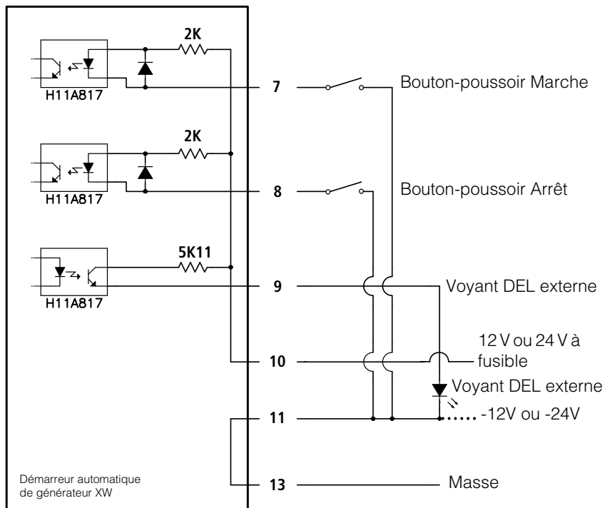
Figure 2-23 Interrupteur externe marche-arrêt et schéma de câblage DEL
