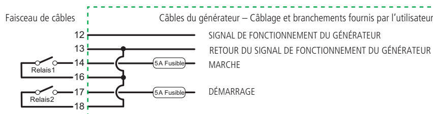
Figure 2-15 Type 8, Schéma de connexions (deux fils)
