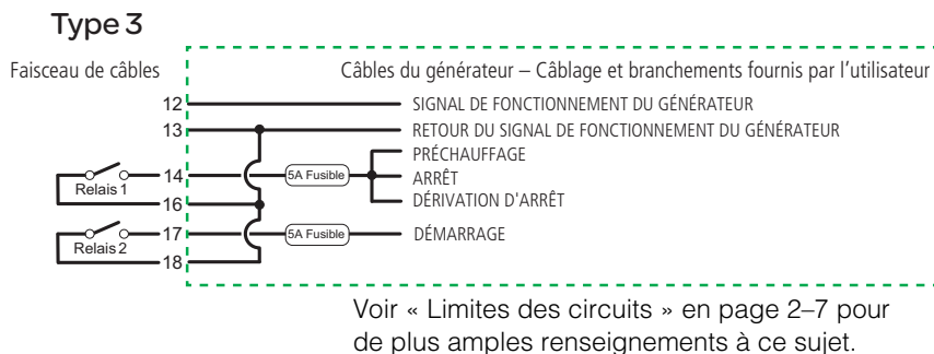
Figure 2-9 Type 3, Schéma de connexions
