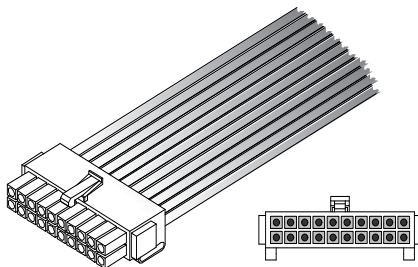
Figure 1-4 Faisceau de câbles
