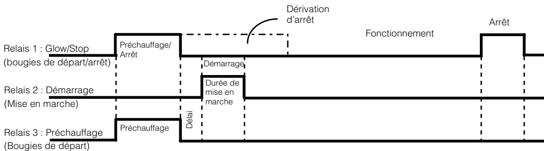
Figure C-9 Schéma de temporisation du mode GlowStop
