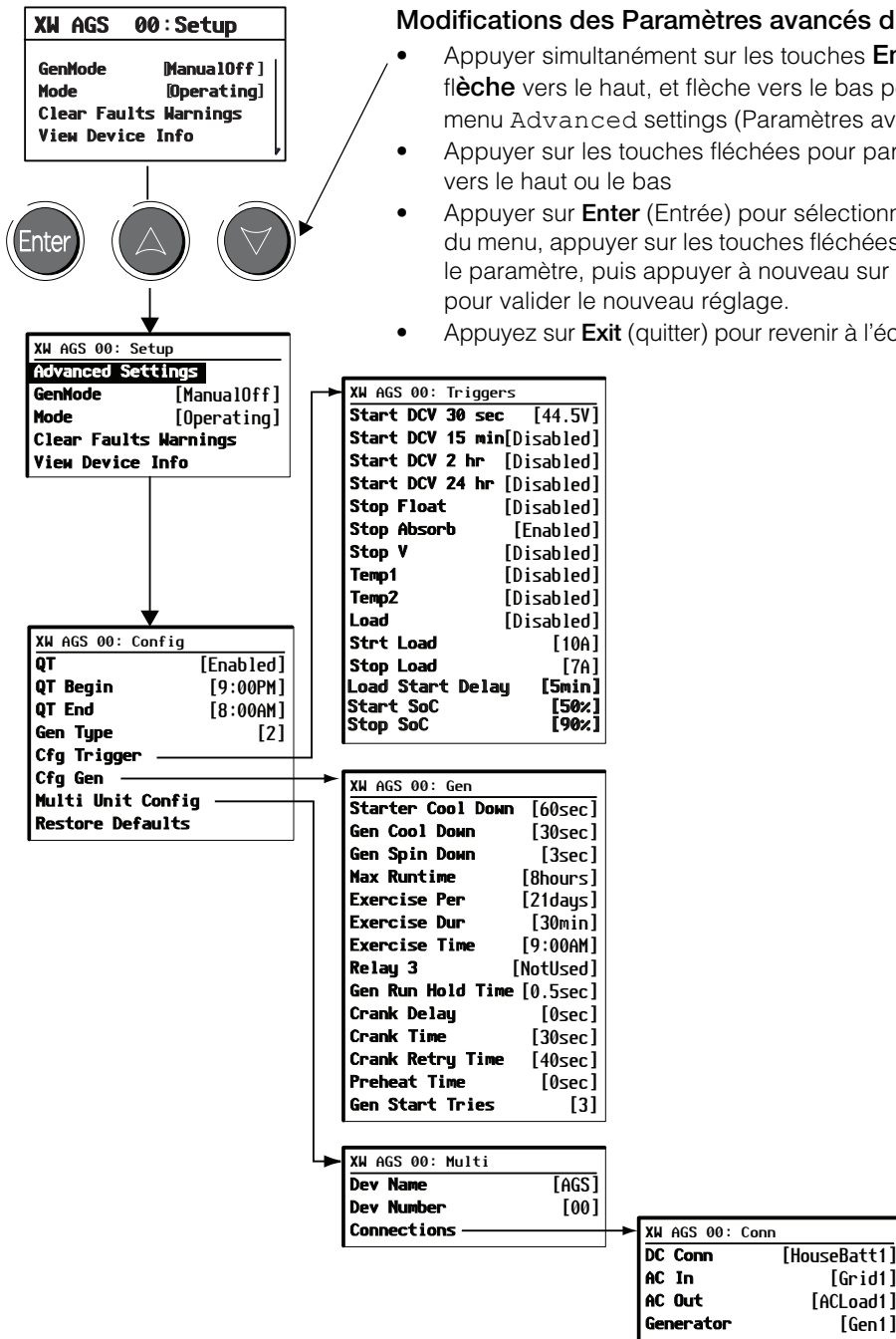
Figure 3-32 Arbrescence des menus des paramètres avancés de l'Conext AGS
