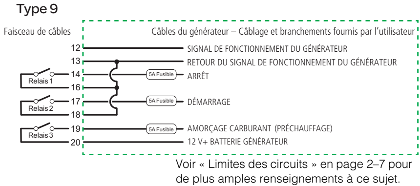
Figure 2-17 Type 9, Schéma de connexions
